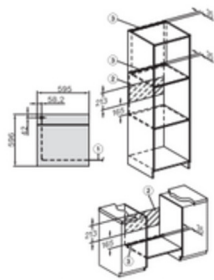
Installation H7000 XL, installation drawing 1) Netzanschlussleitung, L=1500 mm, 2) In diesem Bereich kein Anschluss, 3) Lüftungsausschnitt min. 150 cm 2
