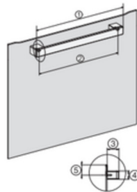
H2465B, H2465BP, H2466B, H2466BP, H2467B, H2467BP, H2468B, H2468BP, H2469B, H2469BP installation drawings EU, 1) 399,6 mm, 2) 360 mm, 3) 45 mm, 4) 31,8 mm, 5) 32,5 mm, EX, 1) 399,6 mm, 2) 360 mm, 3) 45 mm, 4) 31,8 mm, 5) 32,5 mm
