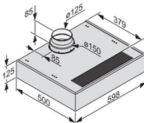
DA 1060, DA 1160, DA 1260 (installation drawing)
